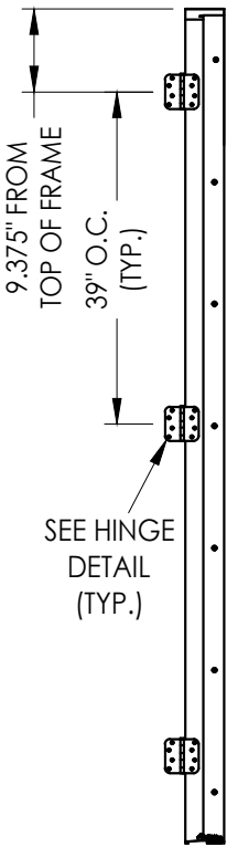
HINGE JAMB
